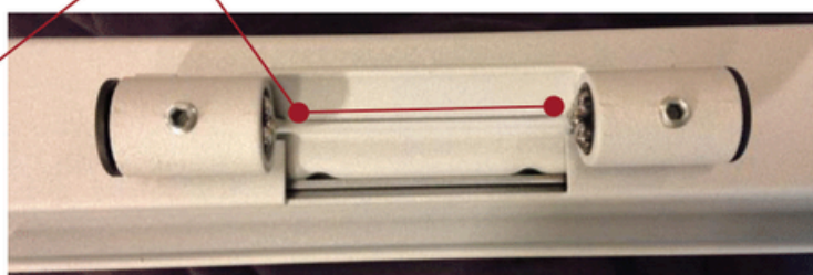
Karmhængsel for bæreløjer (alle kuglerne skal også smøres)
